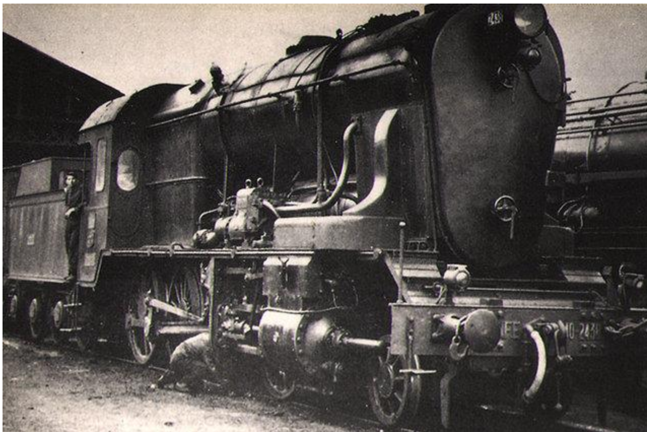
39. Renfe 140-2438, con la caldera Franco-Crosti.
