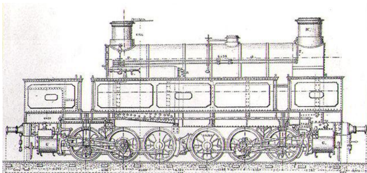
12. Esquema de las locomotoras Norte 801-802.
