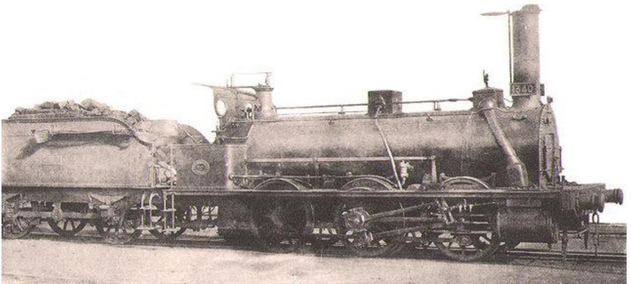
4. Serie 300 (luego serie 1300) caldera vieja.
