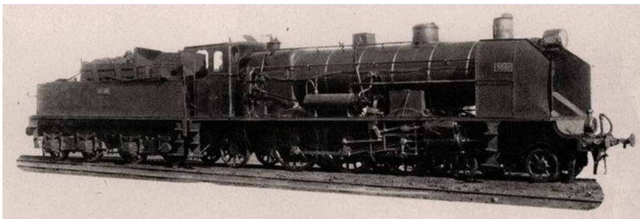
41. Serie 3000, con pantallas levanta humos y precalentador Worthington.
